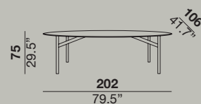
M20_dining table 202 cm
