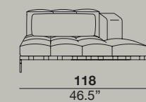
15G_deep 1,5 s left arm 16G_deep 1,5 s right arm
